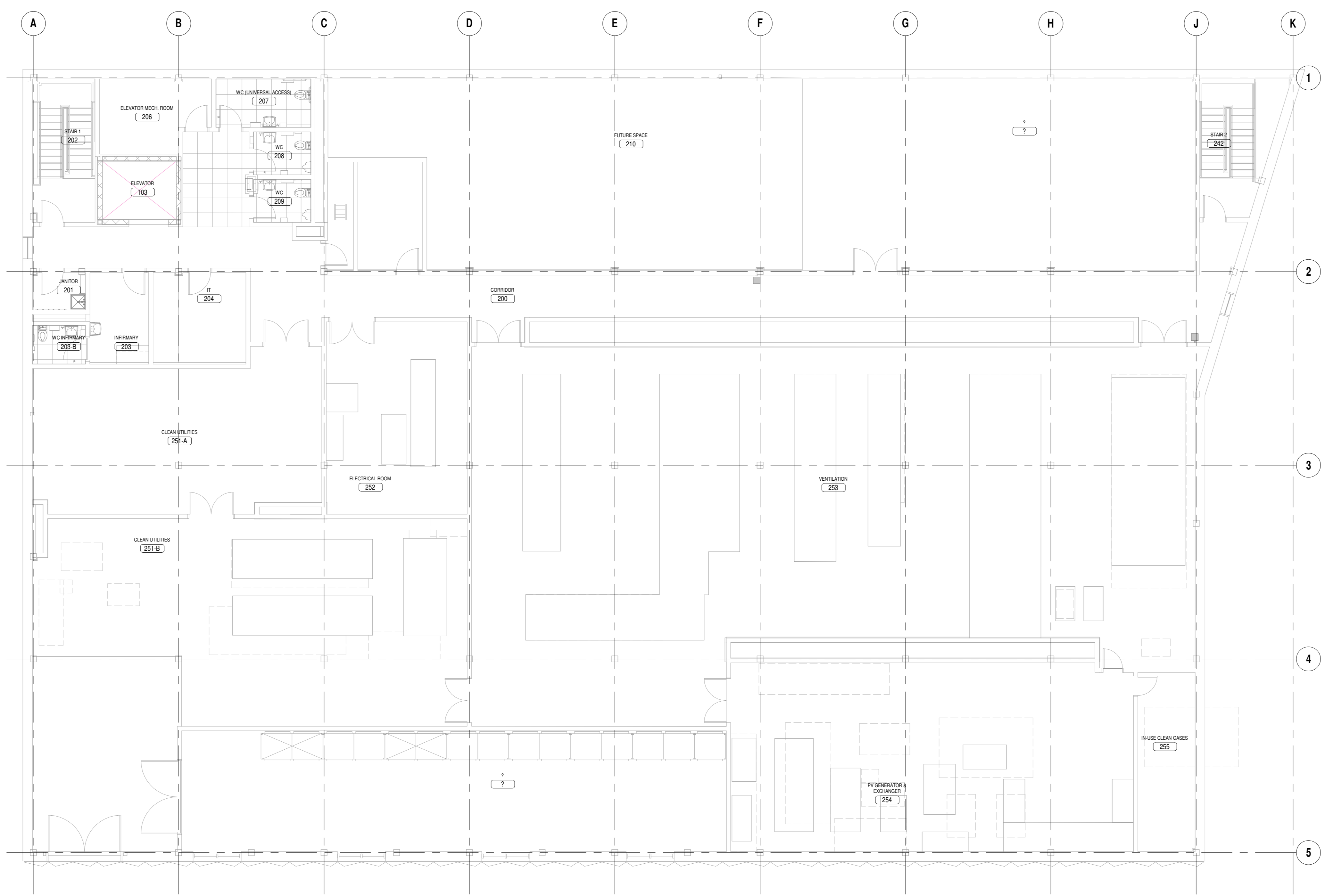
2 2e ÉTAGE - CLASSIFICATION / PRESSURISATION 1 : 100
