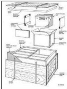
Fig 2. Exemple d'un diagramme d'emballage
