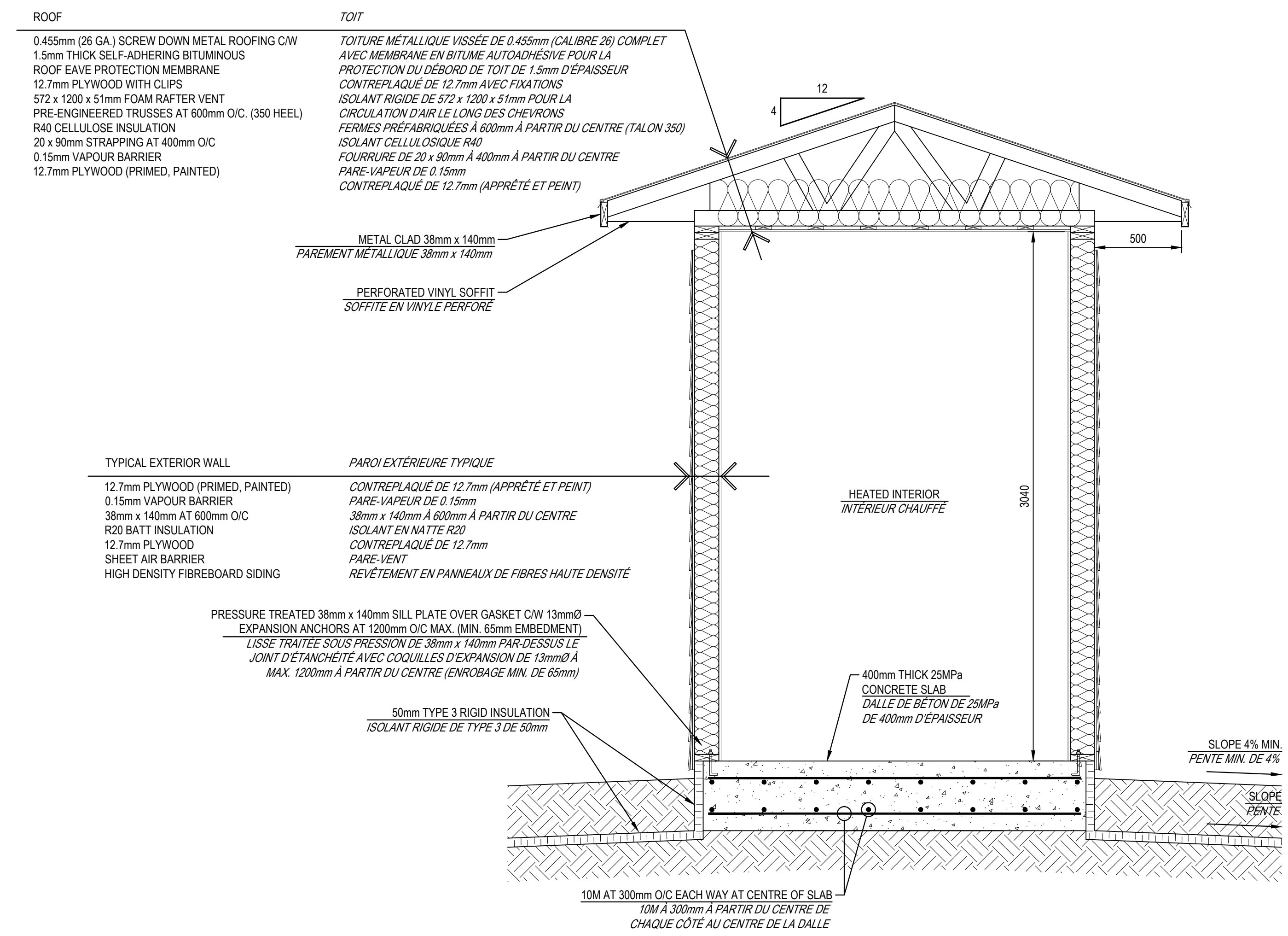
A SERVICE BUILDING 'B' - SECTION E15 BÂTIMENT DE SERVICE 'B' - COUPE TRANSVERSALE SCALE / ÉCHELLE: 1:20
