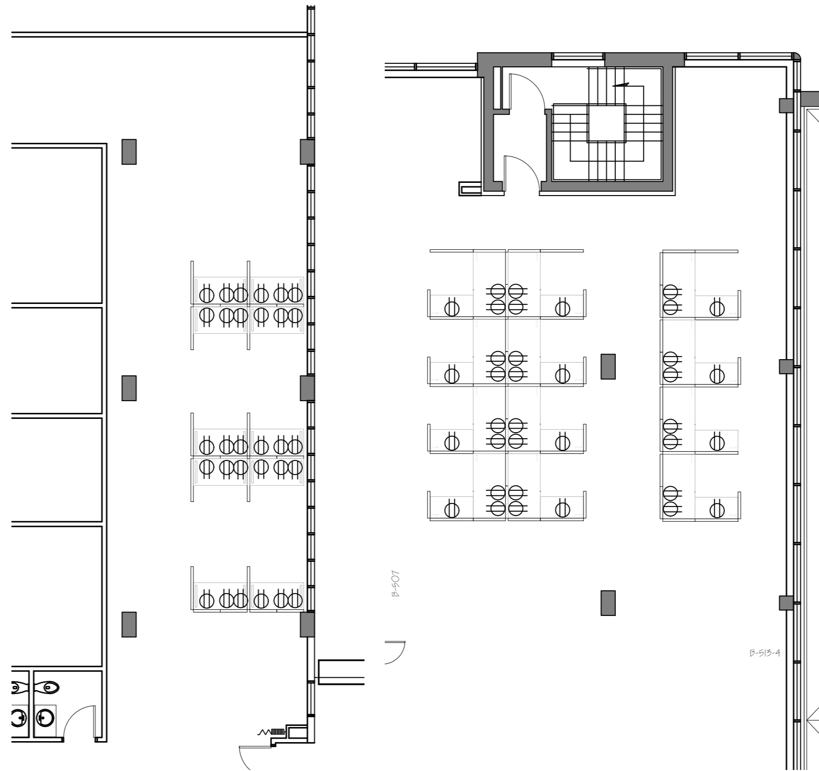
PLAN BESOINS ÉLECTRIQUE ELECTRICAL REQUIREMENTS PLAN
