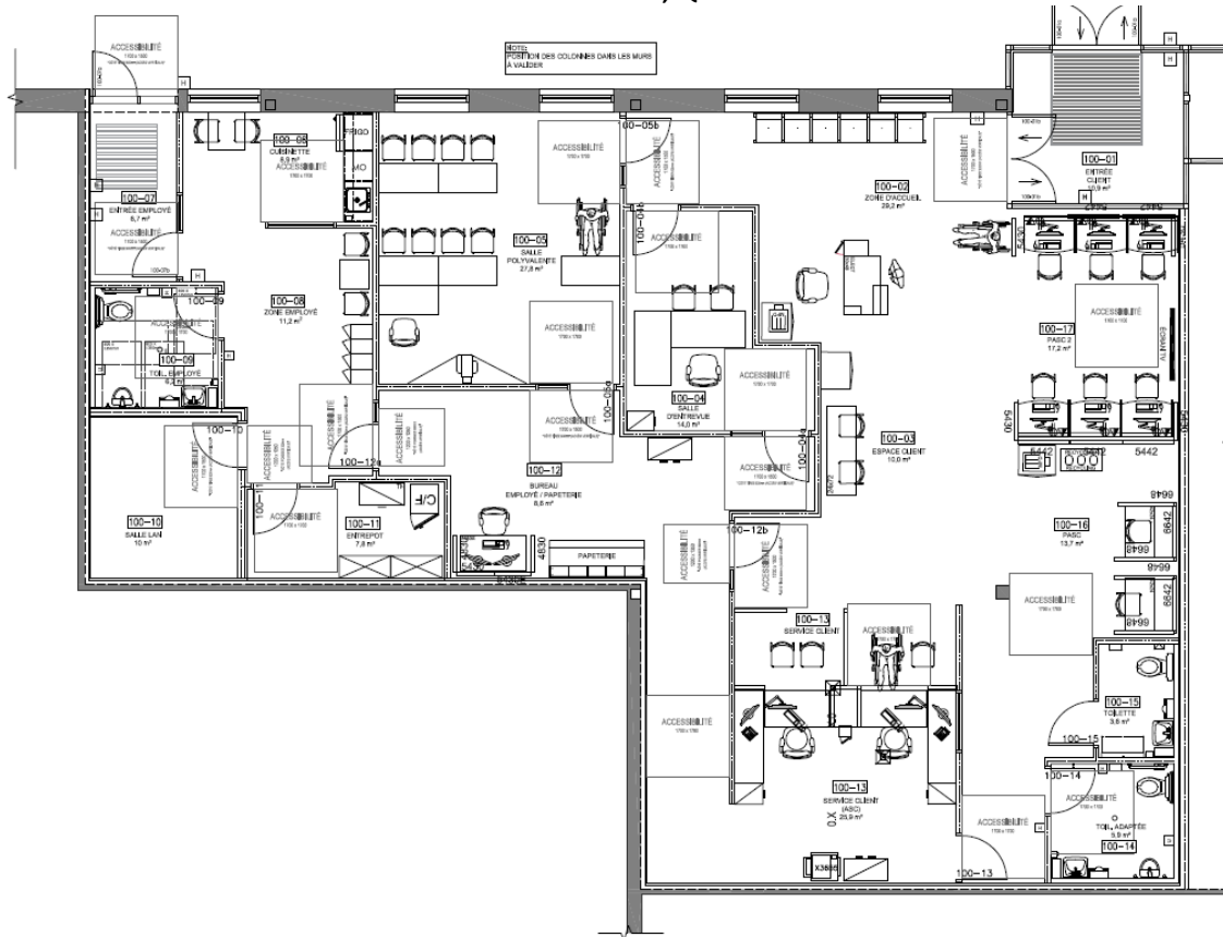
01 PLAN REAMENAGEMENT PLAN DU MOBILIER ÉCHELLE 1/200
